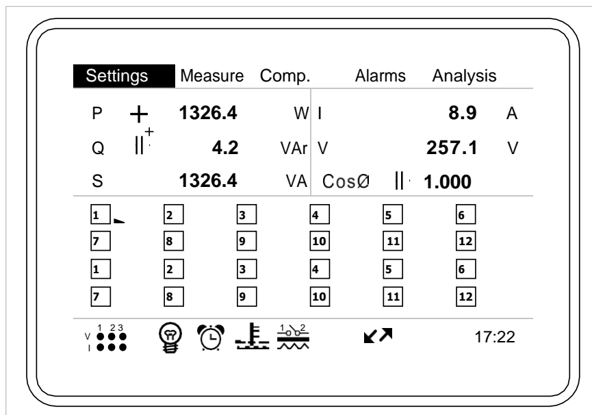
Fig. 1-3 RAPIDUS con 24 RELÉS
