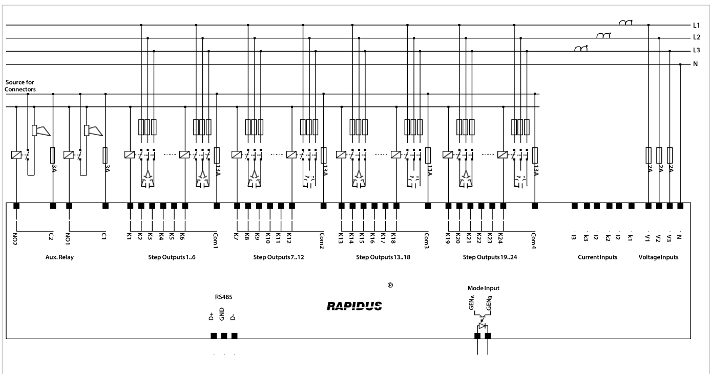
Fig. 2-7 Diagrama de conexión Rapidus (24 Steps)
