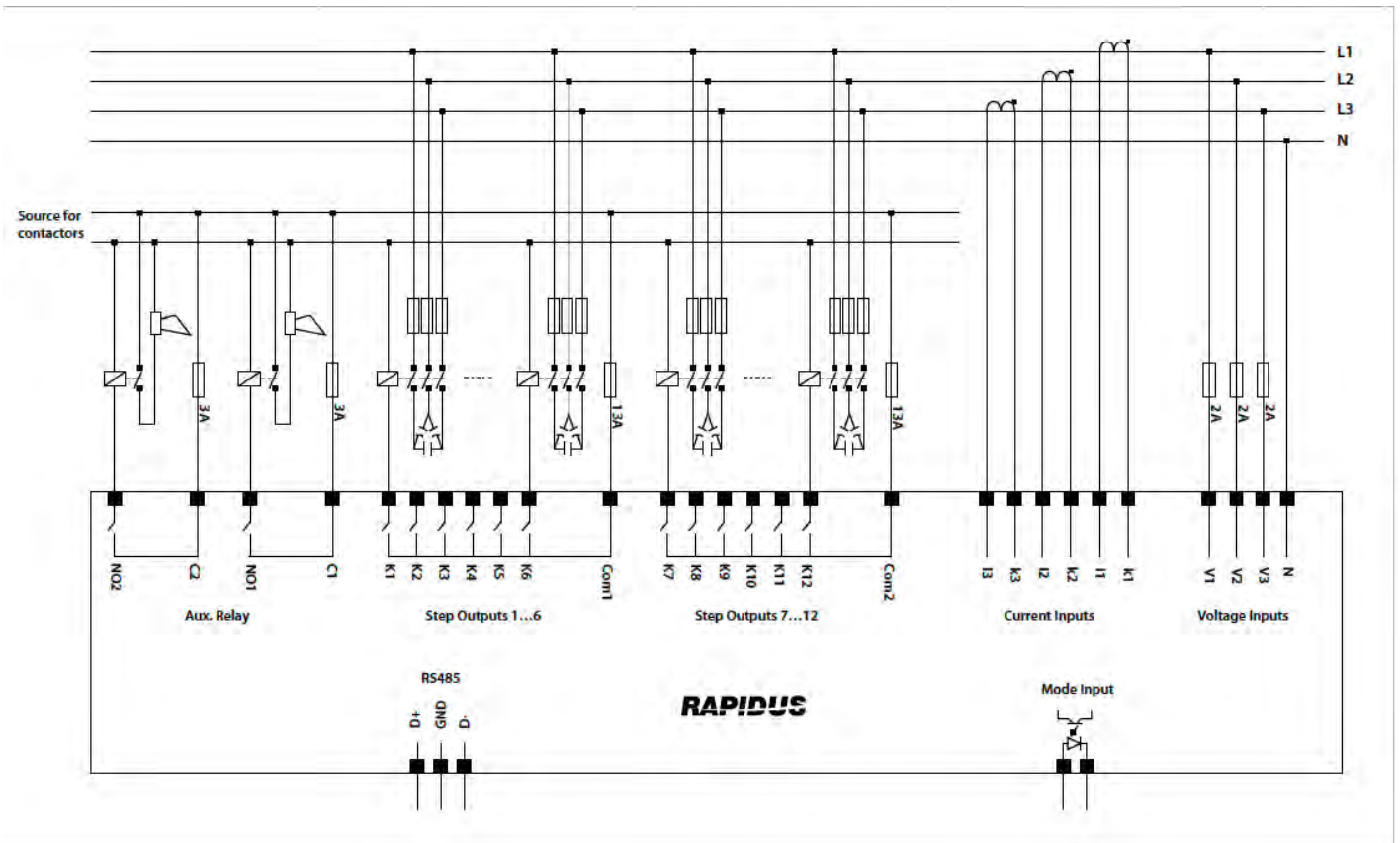
Fig. 2-6 Diagrama de conexión RAPIDUS (12 Steps)
